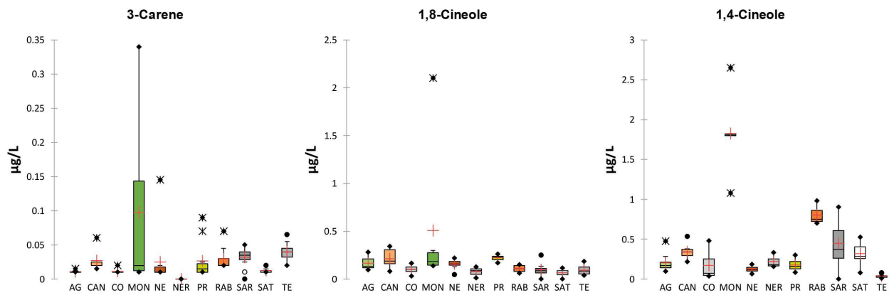
FIGURE 2. Concentration of the bicyclic monoterpene alcohols 3-carene, 1,8-cineole and 1,4-cineole in the different wine variety AG (Aglianico), CAN (Cannonau), CO (Corvina), MON (Montepulciano), NE (Nebbiolo), NER (Nerello Mascalese), PR (Primitivo), RAB (Raboso) SAR (Sangiovese di Romagna), SAT (Sangiovese di Toscana) and TE (Teroldego).
