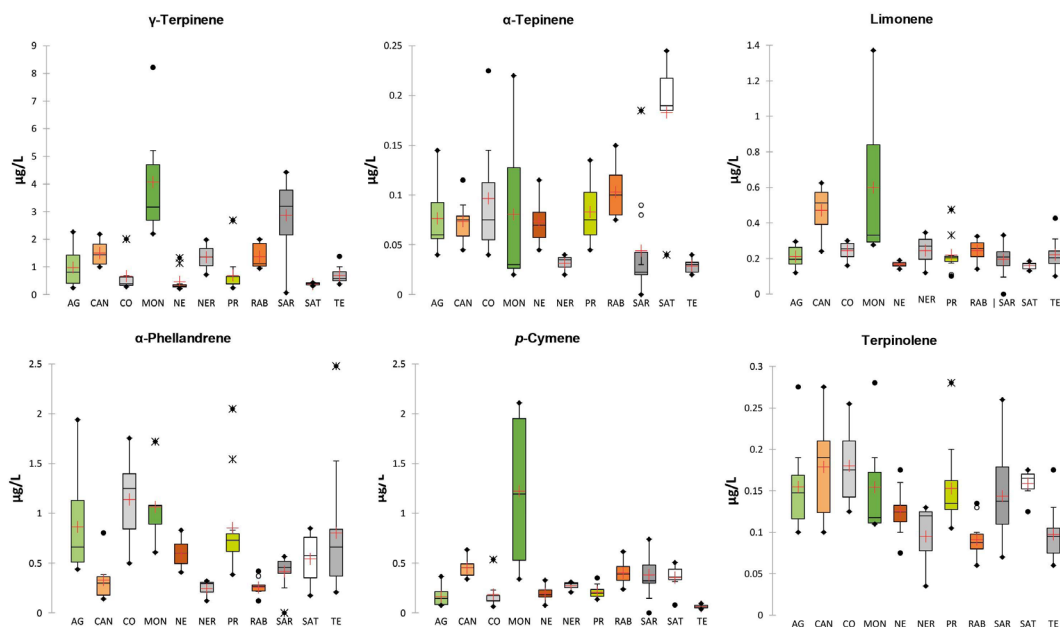
FIGURE 3. Concentration of the cyclic monoterpene alcohols \gamma -terpinene, \alpha -terpinene, limonene, \alpha -phellandrene, p -cymene and terpinolene in the different wine variety AG (Aglianico), CAN (Cannonau), CO (Corvina), MON (Montepulciano), NE (Nebbiolo), NER (Nerello Mascalese), PR (Primitivo), RAB (Raboso) SAR (Sangiovese di Romagna), SAT (Sangiovese di Toscana) and TE (Teroldego).
