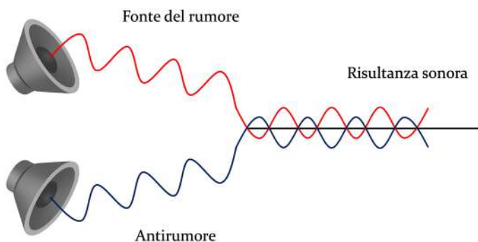
Figura – Schema di funzionamento dell’antirumore e dell’interferenza distruttiva.
