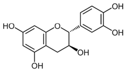
(+)-Catechin (CA)
