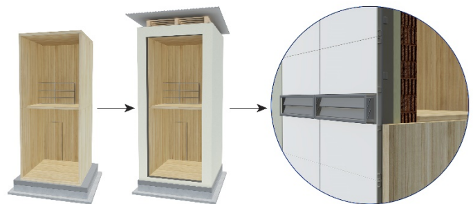
Figura 2 - Render delle fasi principali per la costruzione degli edifici test e a destra il dettaglio schematizzato della facciata ventilata.
