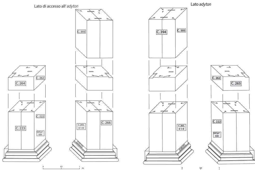
FIGG. 7-8. Ricostruzione dei pilastri di accesso all'adyton del tempio di Apollo. Disegno di Mariagrazia Divincenzo.
