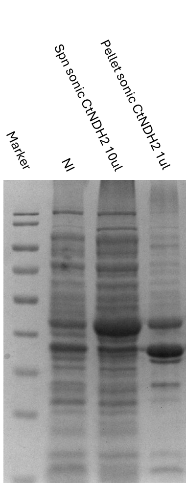
SDS-PAGE lisato sonificatore C41(DE3) + CtNDH2
