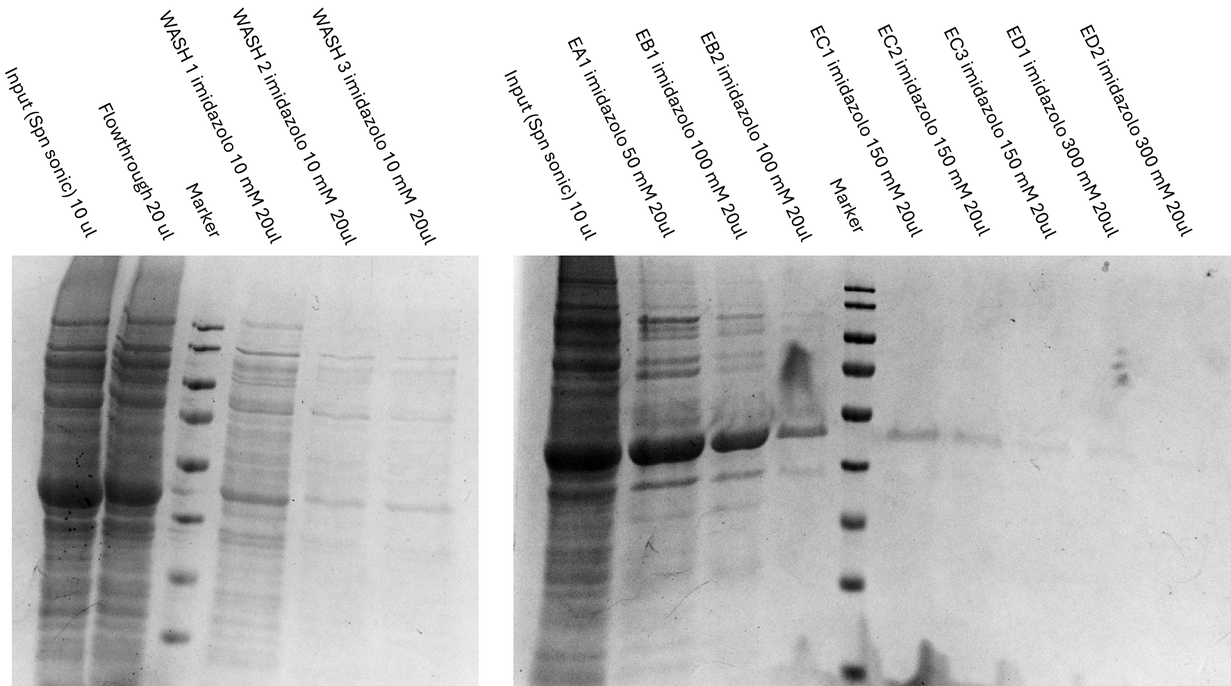
SDS-PAGE purificazione CtNDH2 tramite His-trap da spn sonificatore
