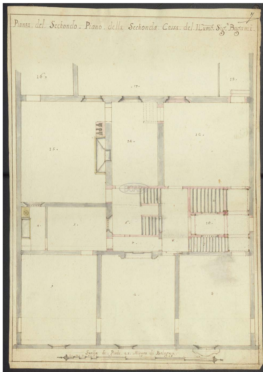
5. [Giacomo Galli]: Pianta del secondo piano della seconda casa dell' Illustrissimo Signor Bugami , 1708? Bologna, Biblioteca Comunale dell' Archiginnasio, Ms. B4357, n. 7
