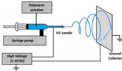
Fig. 2 Electrospinning apparatus
