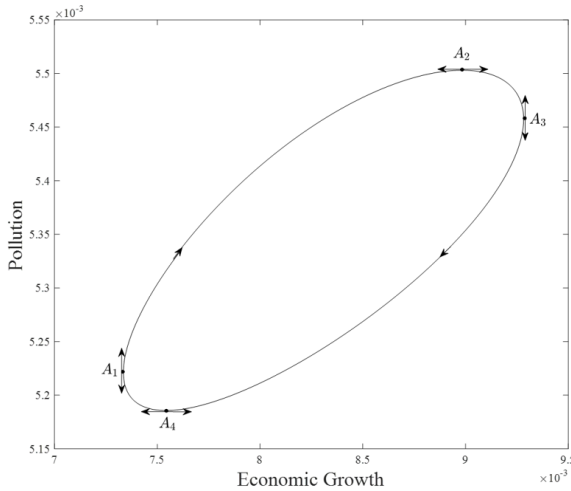
7a. \pi_k = 0.5691
