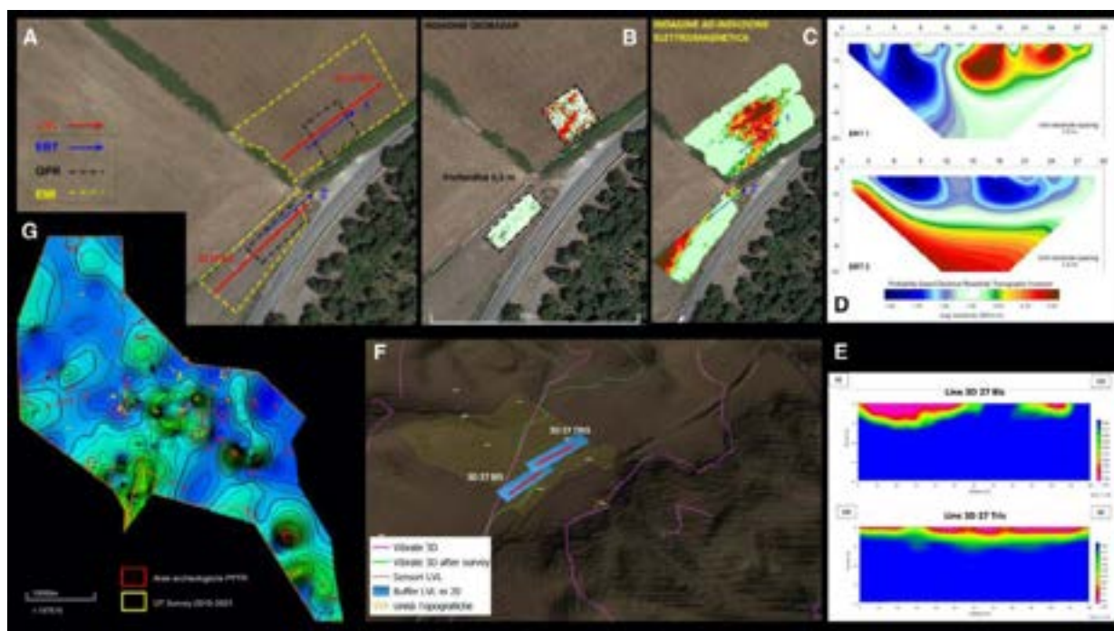
Figura 3 - Sicilia sudorientale, A) Monterosso Almo, prospezioni geofisiche eseguite in contrada Muraglie, (B-F), indagini ad induzione elettromagnetica (EMI), tratteggio giallo, circa 2800 m 2 a Nord e circa 1000 m 2 a Sud; tratteggio nero, georadar (GPR) 400 m 2 a nord e 300 m 2 a sud, frecce blu; tomografie elettriche di resistività (ERT) (elab. M. Cozzolino, V. Gentile); G) Monti Iblei, modello velocità delle onde P ottenuto mediante interpolazione velocità delle litologie affioranti (elab. S. Montalbano)
