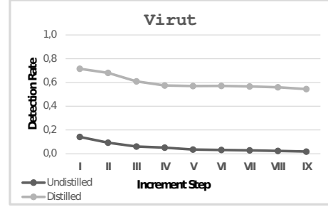
(d) Group 4a: Duration & Src_Bytes & Dst_Bytes & Tot_Pkts
