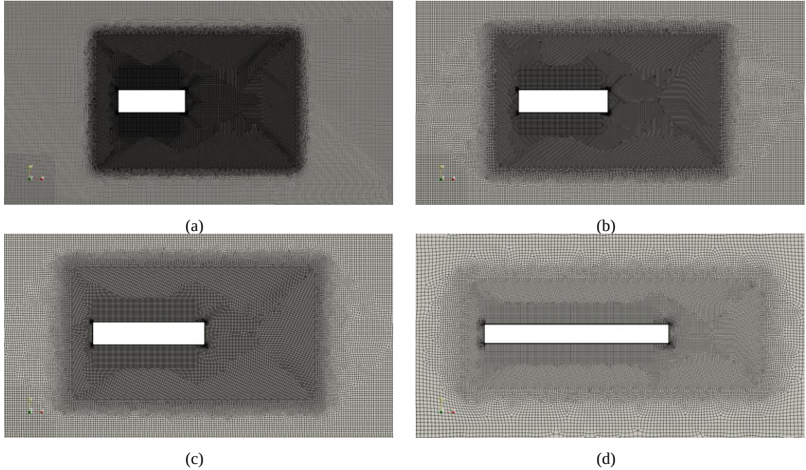
Figure 3. Detailed meshes around rectangular cylinders: (a) R3 ; (b) R4 ; (c) R5 ; (d) R10 .
